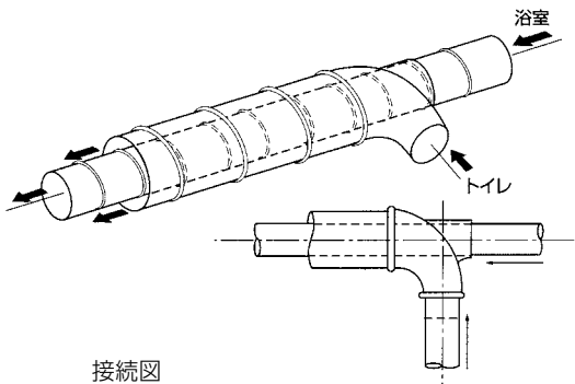
接続図
