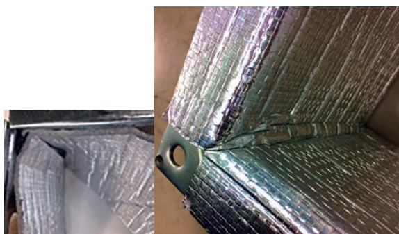
図4. 組立て後のコーナー部
