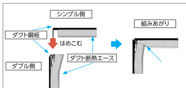
図5. 断熱ダクト断面図
